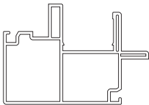
FRONT JAMB BV686801
